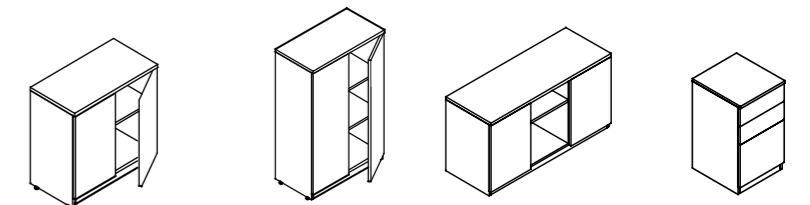
1. V-S 7575: W 750 x D 400 x H 750 2. V-S 9075: W 900 x D 400 x H 750
